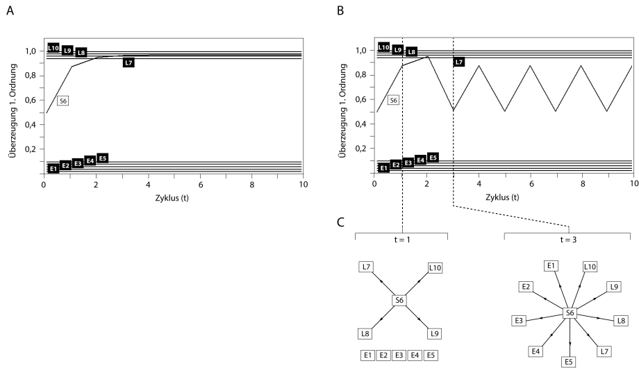
Abbildung 5: Meinungsdynamik der Überzeugungen erster Ordnung (A, B) sowie die durch die Überzeugungen zweiter Ordnung bestimmten Vertrauensbeziehungen zu den angegebenen Zyklen t für die in B dargestellte Simulation (C). Eine in der Abbildung durch einen Pfeil dargestellte Vertrauensbeziehung ergibt sich, wenn eine Person eine andere für epistemisch kompetent hält und zudem das Kohärenzkriterium erfüllt wird.
